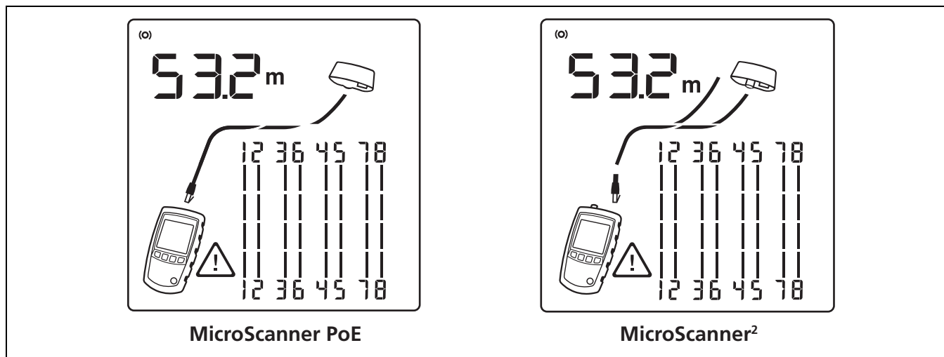
Figura 14. Detectada derivação em paralelo
