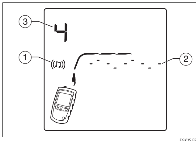
Figura 35. Tela do modo de gerador de tom analógico
