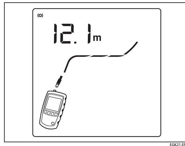
Figura 24. Abertura em cabeamento coaxial (MicroScanner 2 )
