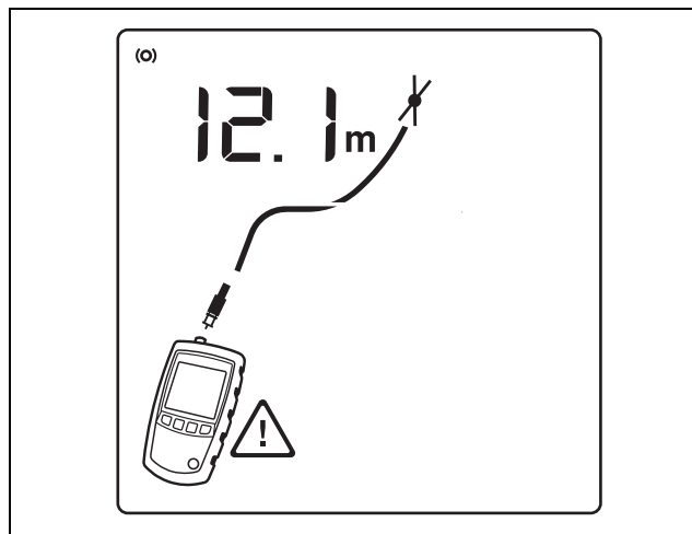
Figura 25. Curto em cabeamento coaxial (MicroScanner²)
