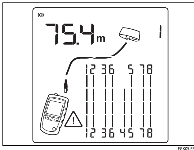
Figura 8. Abertura em cabeamento de par trançado
