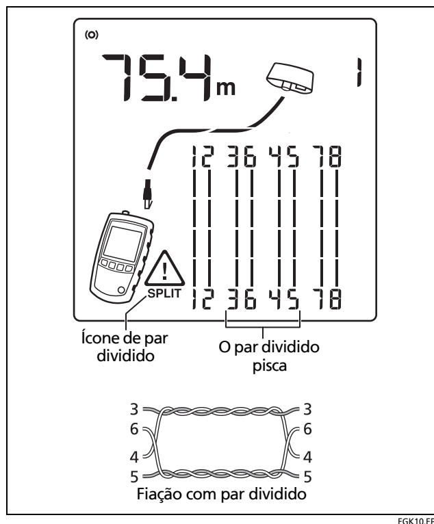
Figura 12. Par dividido
