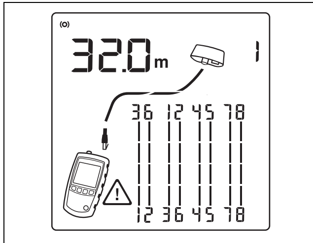
Figura 11. Pares cruzados
