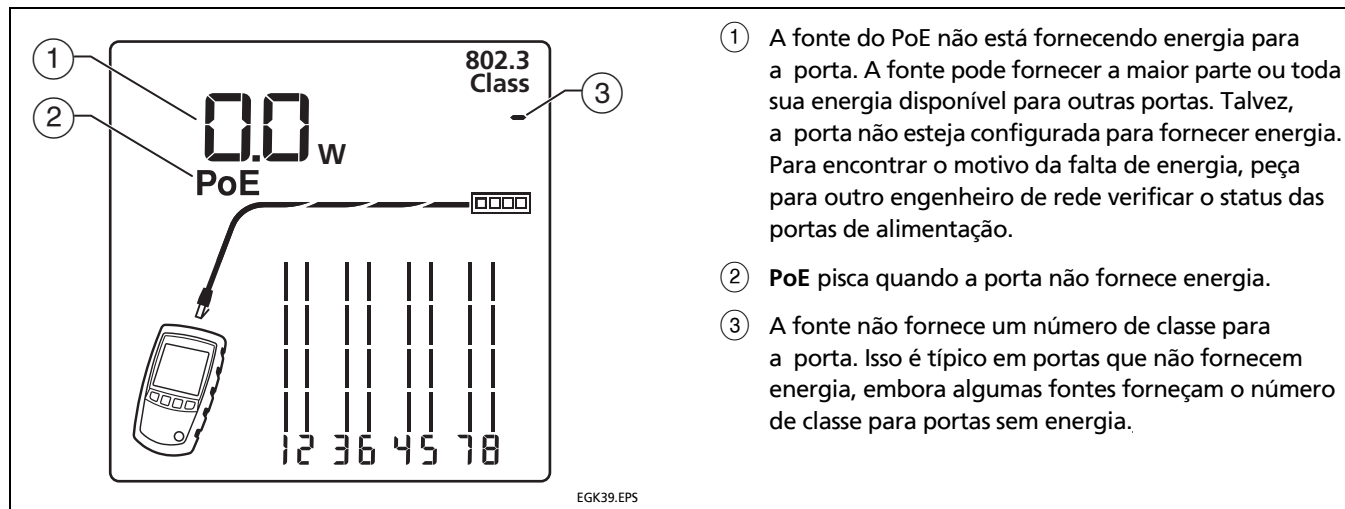
Figura 31. Porta PoE que exibe 0.0 W
